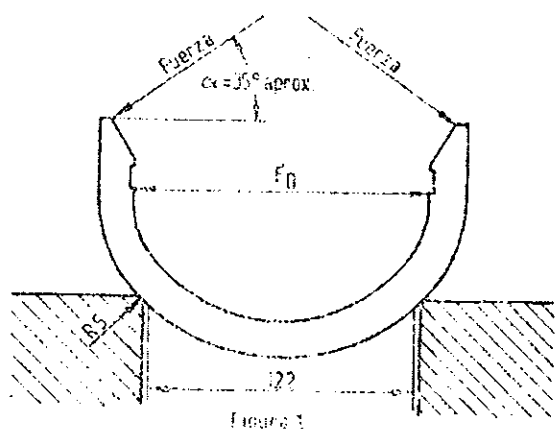
Figura 1 Ensayo de deformación inicial
