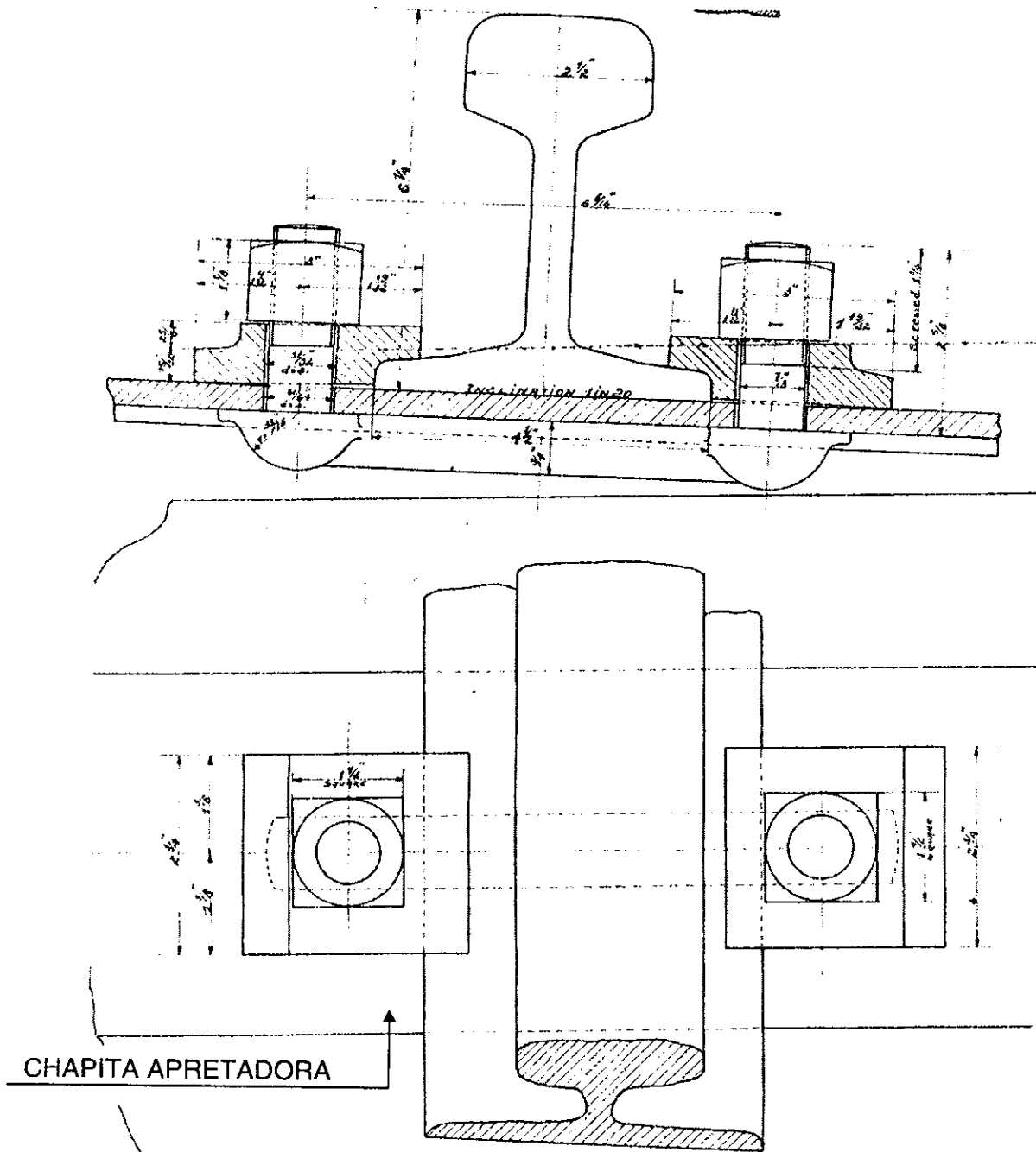
FIGURA 19 CHAPITAS APRETADORAS (CLIPS)
